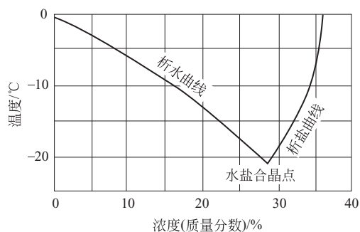
图 10.3 氯化钠水溶液结晶曲线
