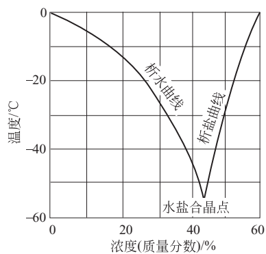
图 10.4 氯化钙水溶液结晶曲线
