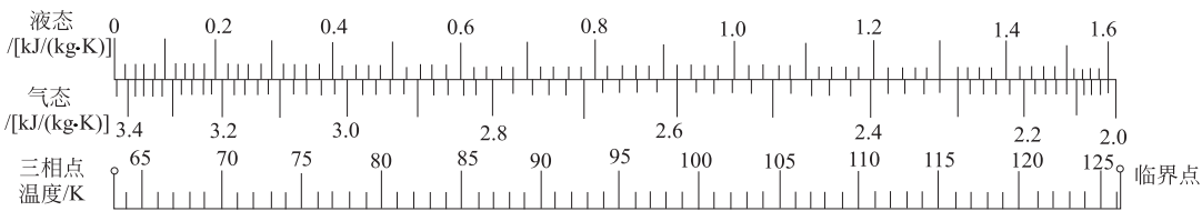
图 2.17 常压下氮气的比熵
