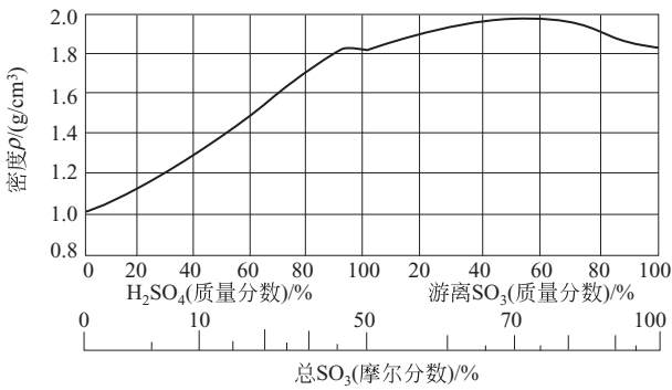
图 5.2 三氧化硫与水混合物的密度 (40℃)
