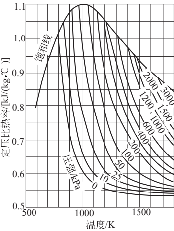
图 4.4 钾蒸气的定压比热容
