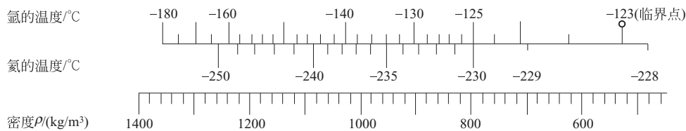
图 2.6 氩和氮液体的密度
